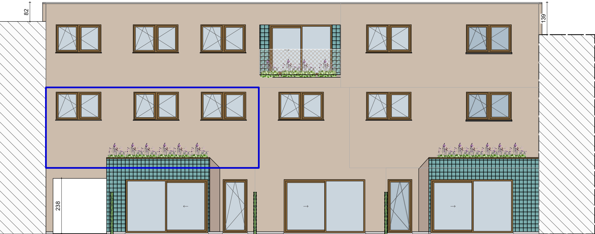
Achtergevel
